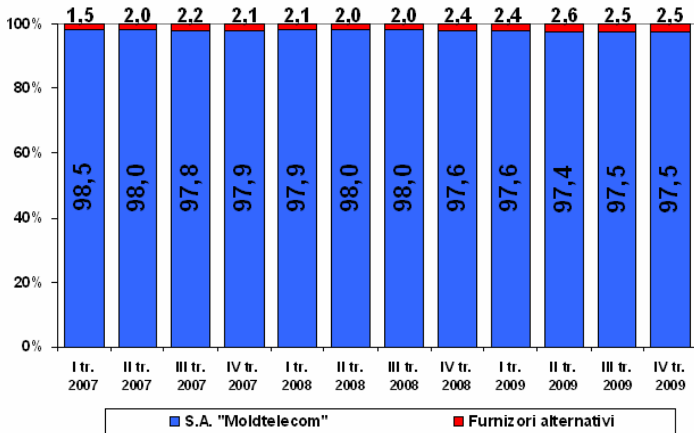
Fig. nr. 4. Structura pieței, în funcție de numărul de abonați
